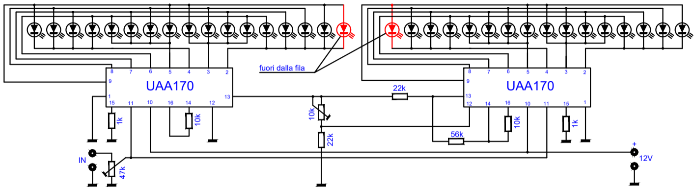
INDICATORE TENSIONE CON FILA DI LED
