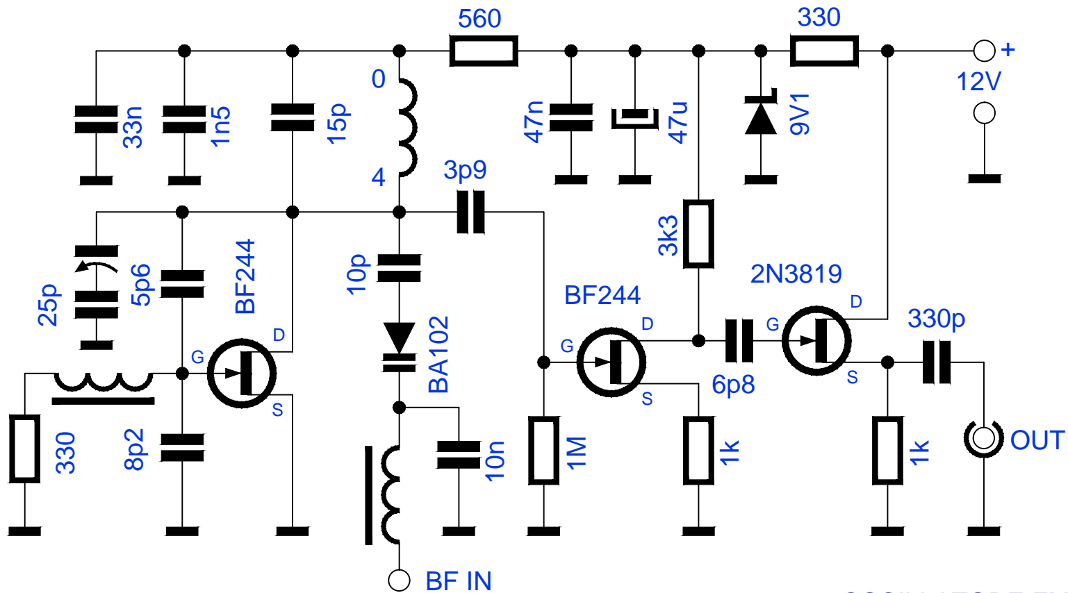
OSCILLATORE FM
