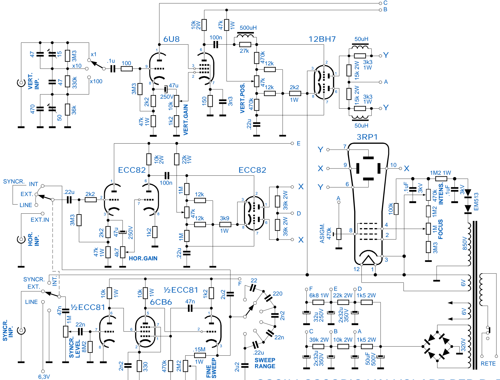
OSCILLOSCOPIO VALVOLARE PER B. F.
