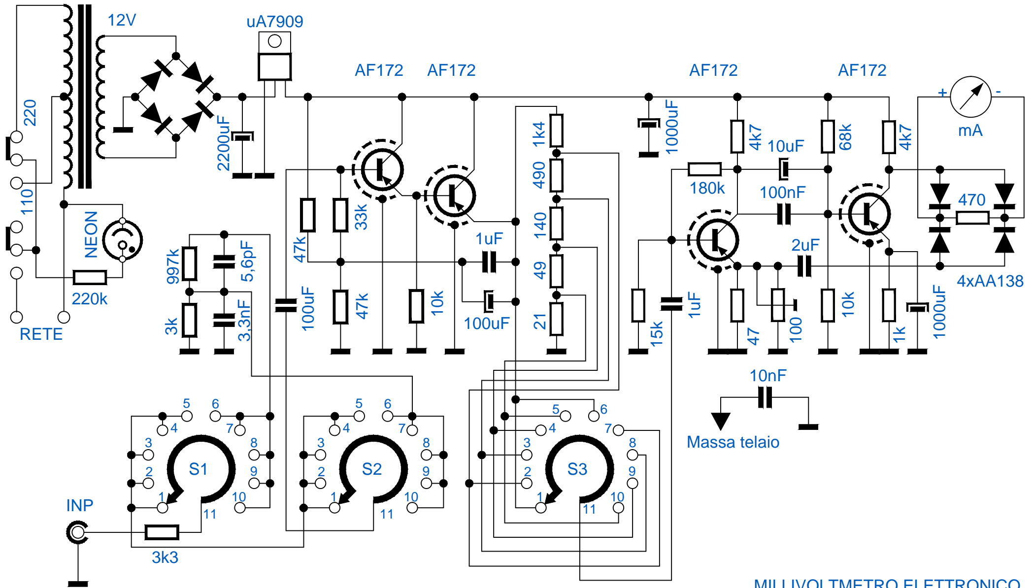
MILLIVOLTMETRO ELETTRONICO
