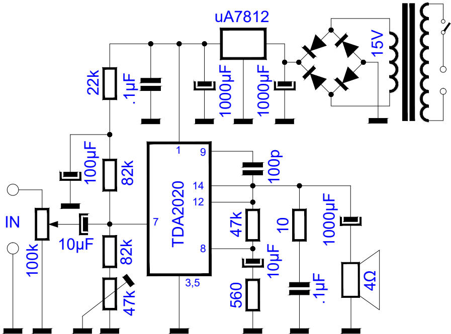
AMPLIFICATORE 4W
