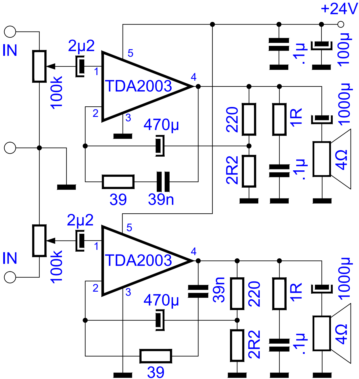
AMPLIFICATORE 10+10W
