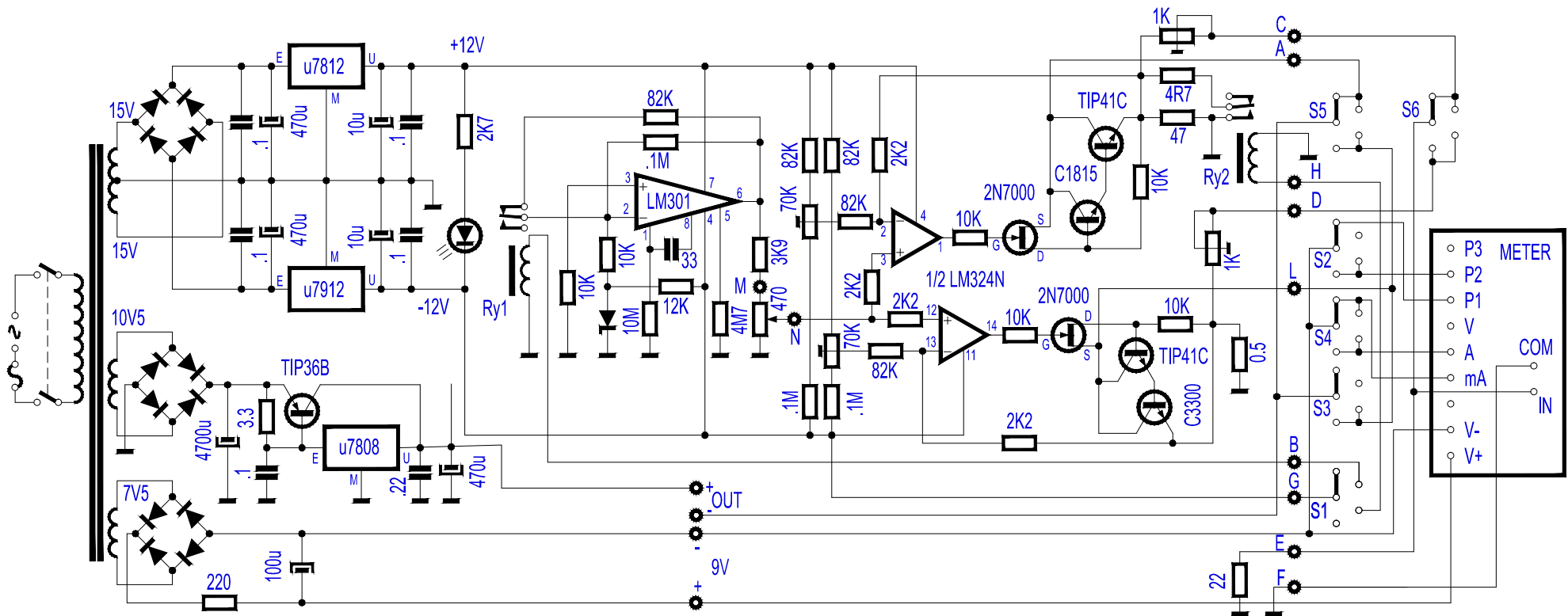
GENERATORE DI CORRENTE COSTANTE
