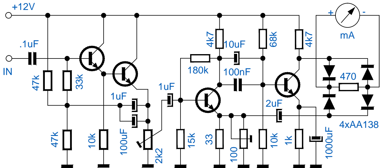
MILLIVOLTMETRO AC
